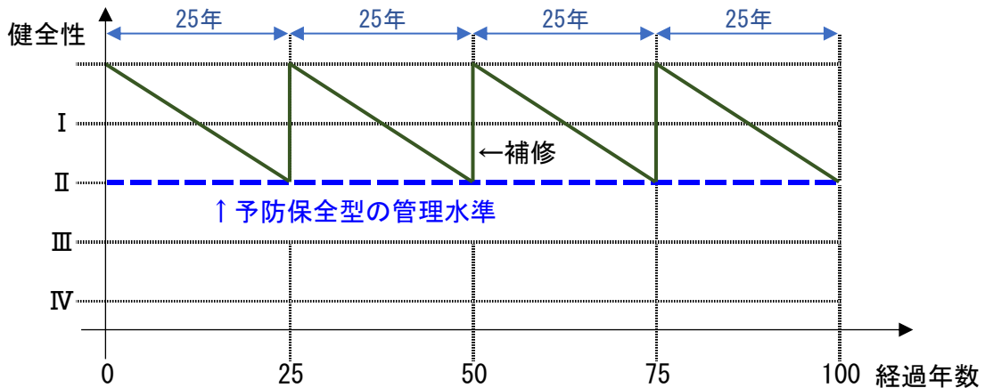
図12.1 対策時期の概念図（予防保全型）
