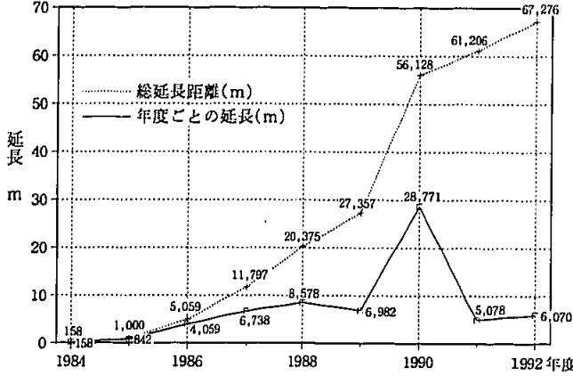
(図二) 下水道管の延長距離 (年度ごと及び総延長)
